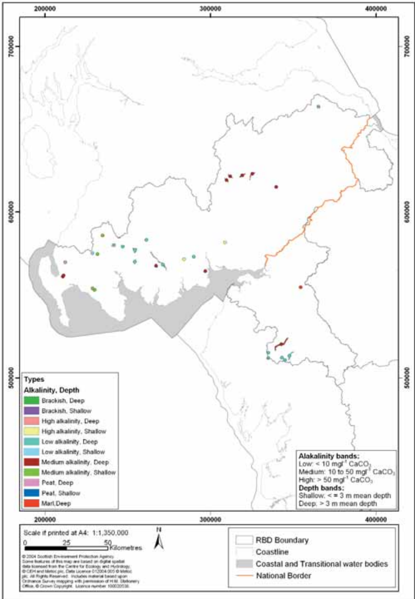
Map 3: Lake types
